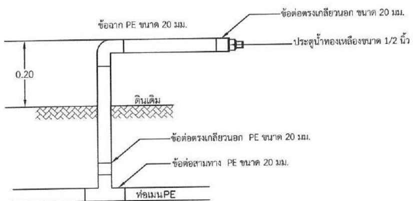
แบบการติดตั้งจุดจ่ายน้ำเข้าบ้าน มาตราส่วน NOT TO SCALE
