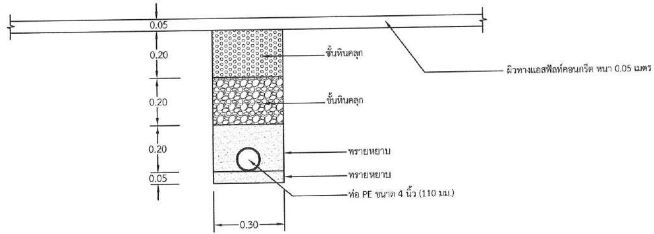
แบบขยายชุดวางท่อผ่านถนนลาดยาง
