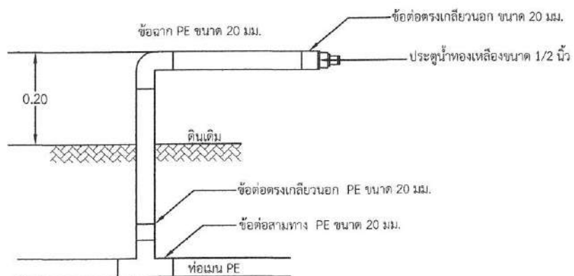
แบบการติดตั้งจุดจ่ายน้ำ มาตราส่วน NOT TO SCALE
